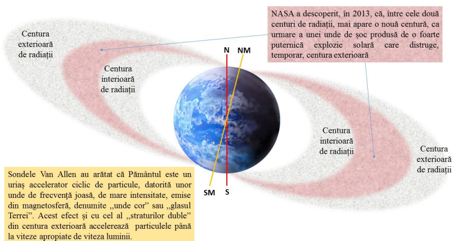
Fig. nr. 1 Centurile de radiații Van Allen 108
